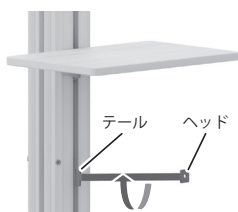
① TUGUCAタテのスリットに、シングルトレー支持金具のテールを差し込み、90度回転させます。
